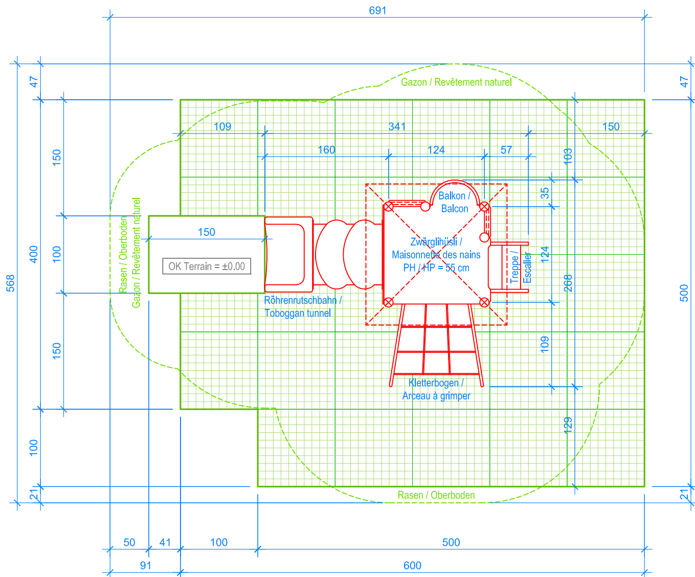
GRUNDRISS / PLAN 1:50
