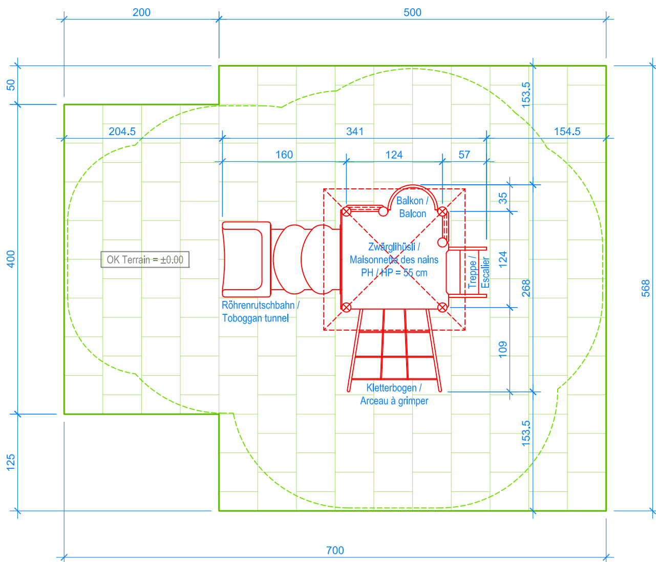
GRUNDRISS / PLAN 1:50
