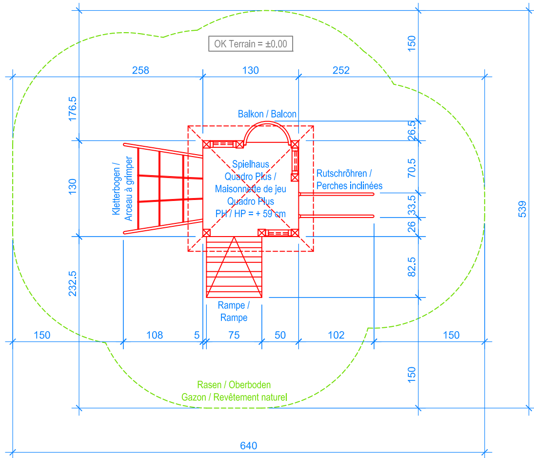
GRUNDRISS / PLAN 1:50
