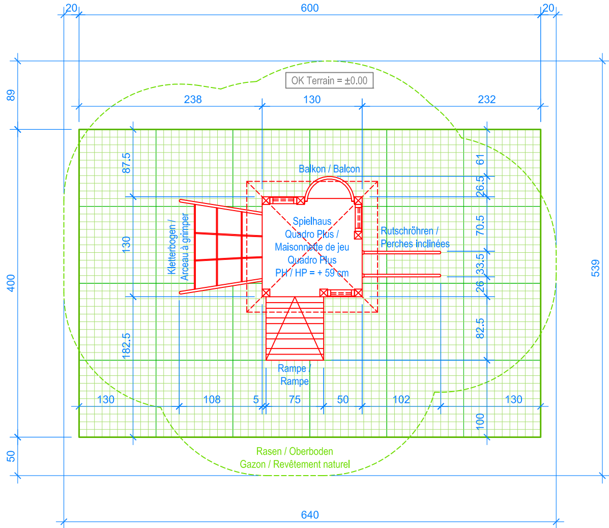
GRUNDRISS / PLAN 1:50
