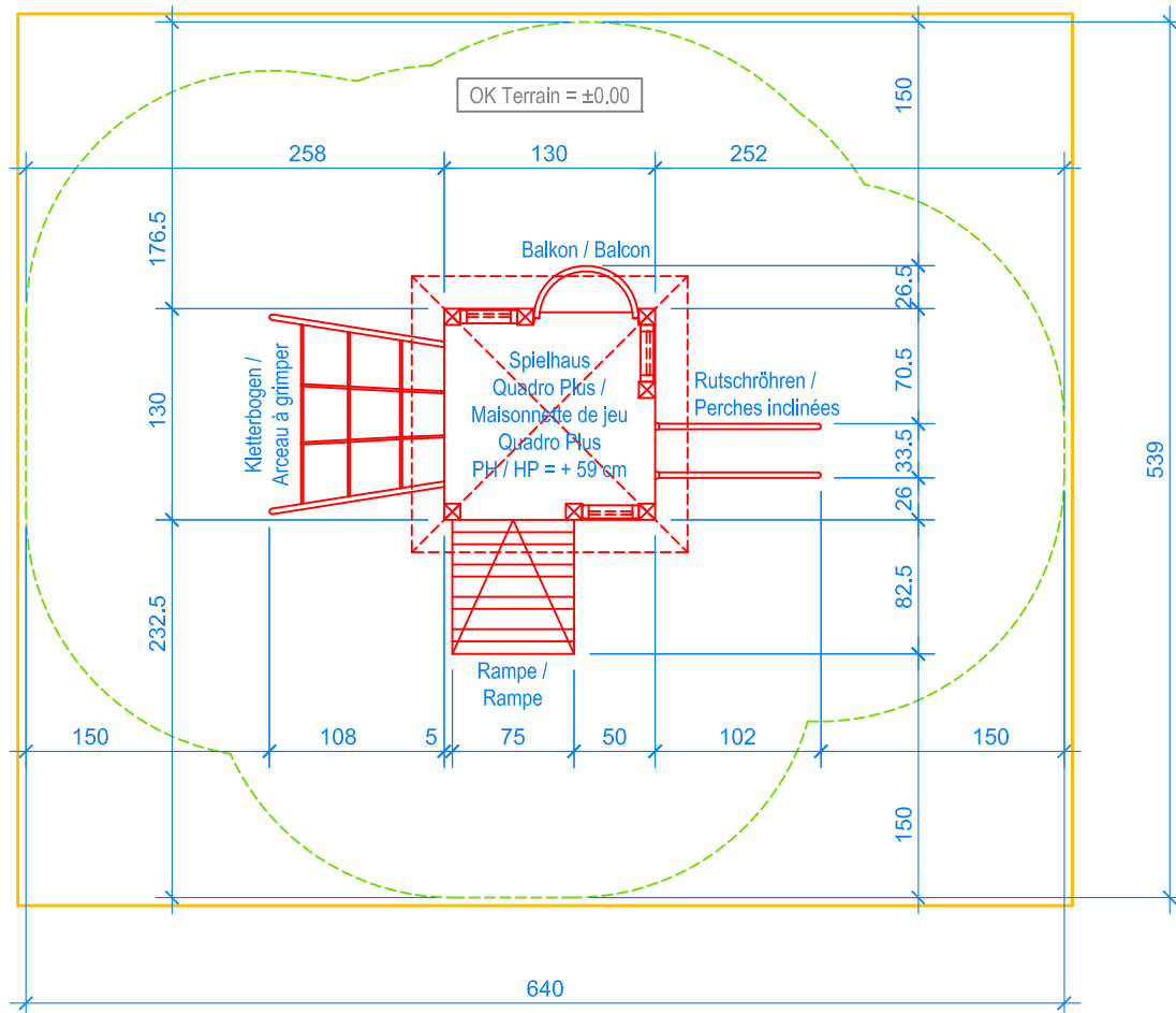
GRUNDRISS / PLAN 1:50
