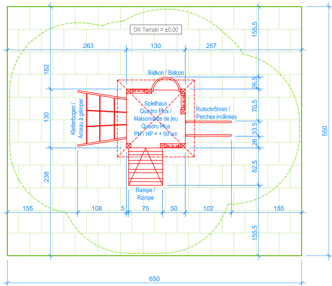
GRUNDRISS / PLAN 1:50
