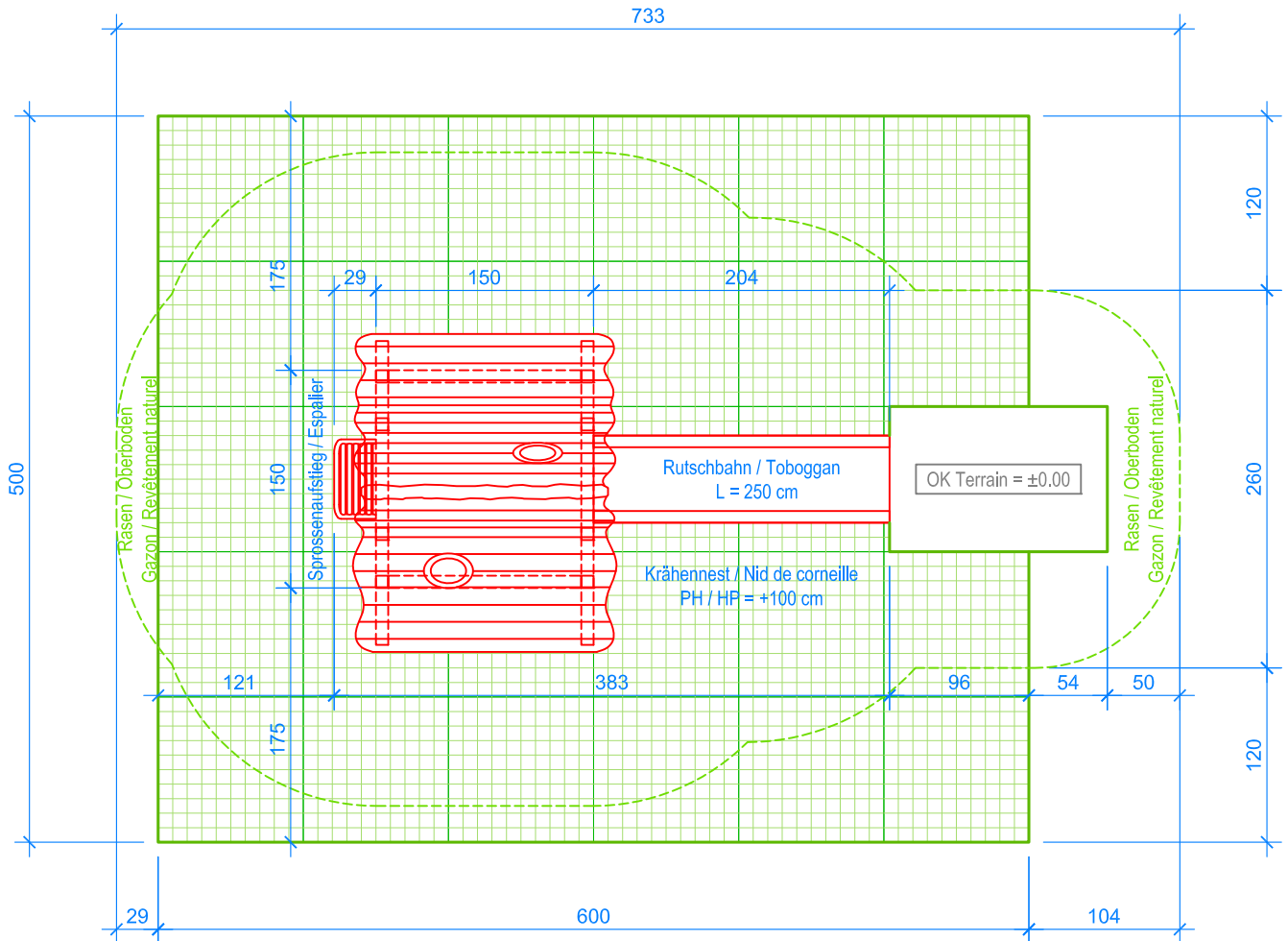
GRUNDRISS / PLAN 1:50
