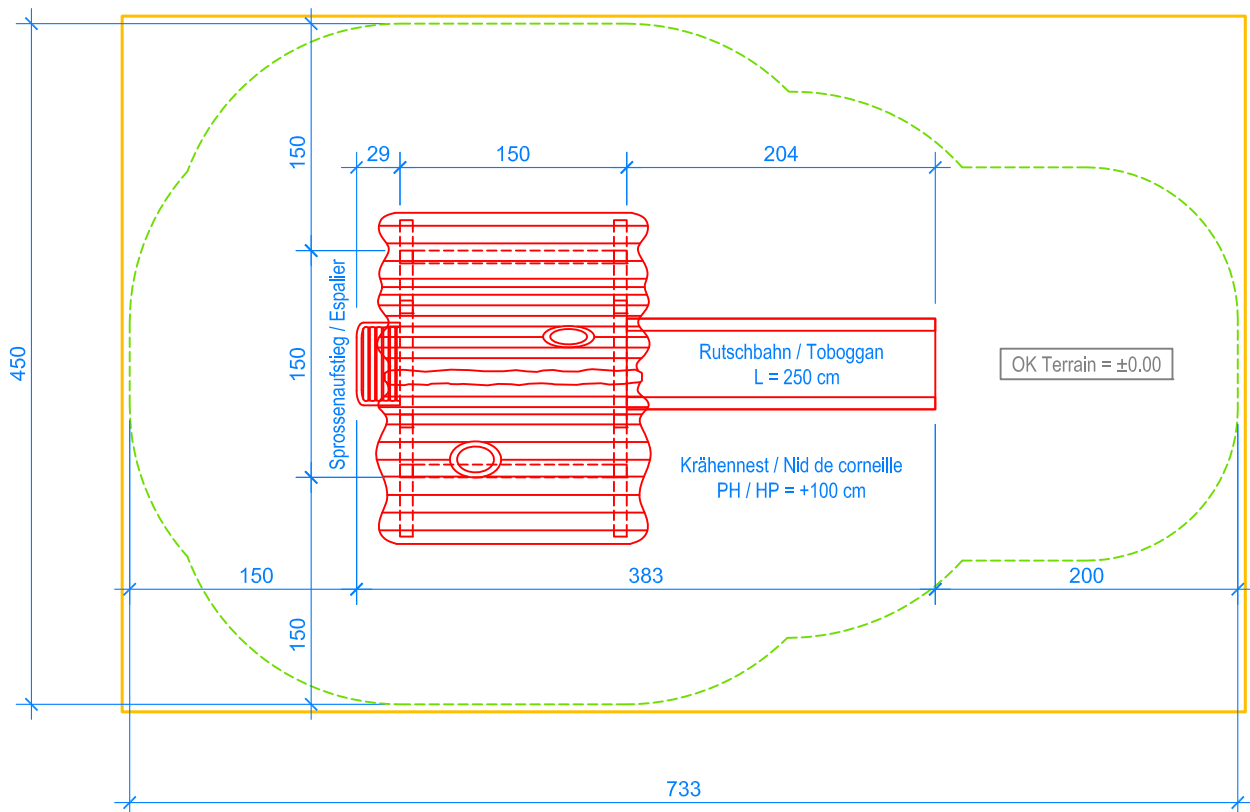
GRUNDRISS / PLAN 1:50
