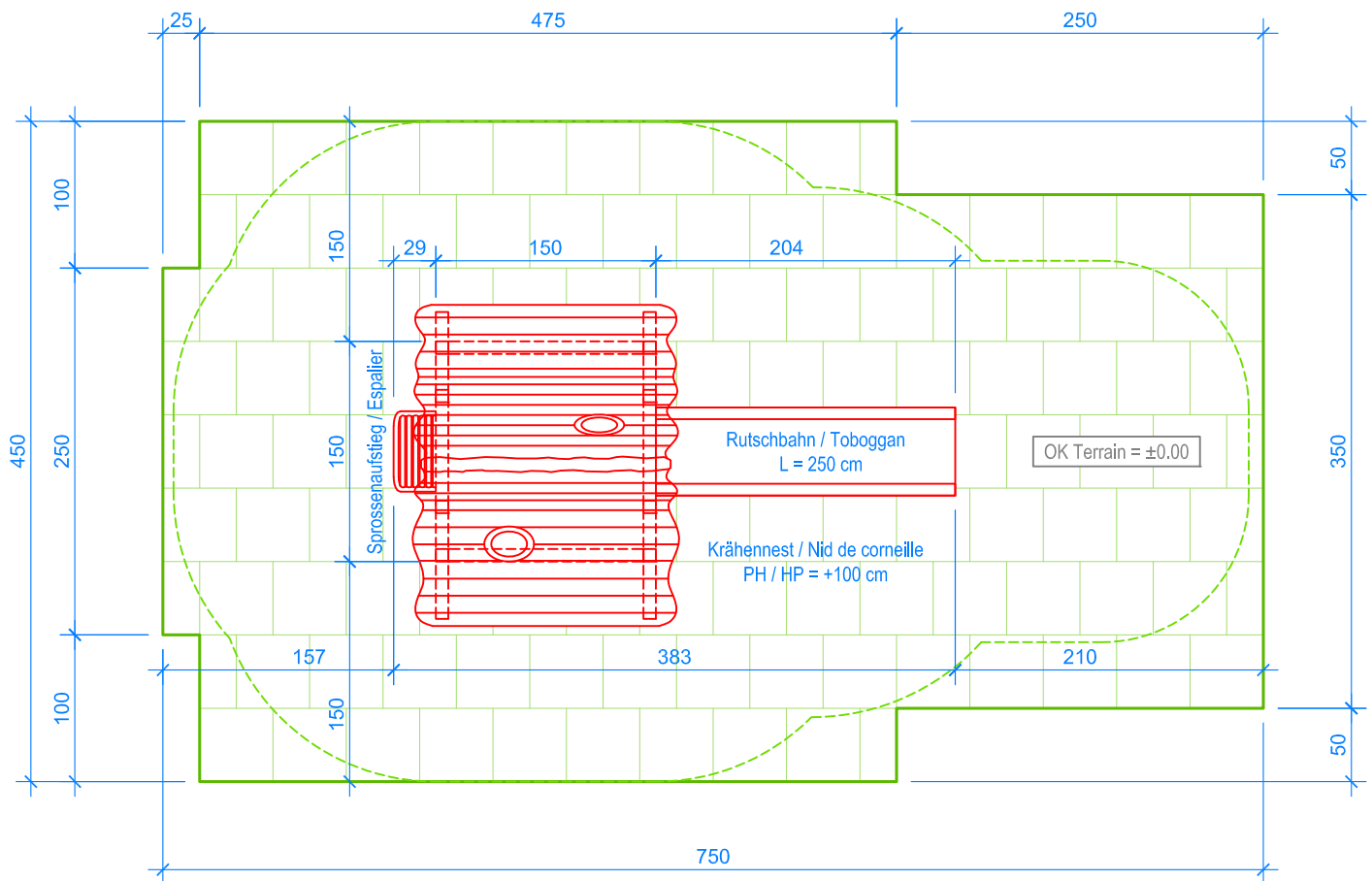
GRUNDRISS / PLAN 1:50
