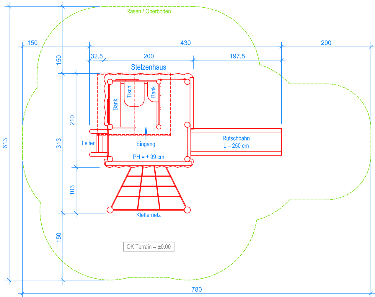
GRUNDRISS 1:50
