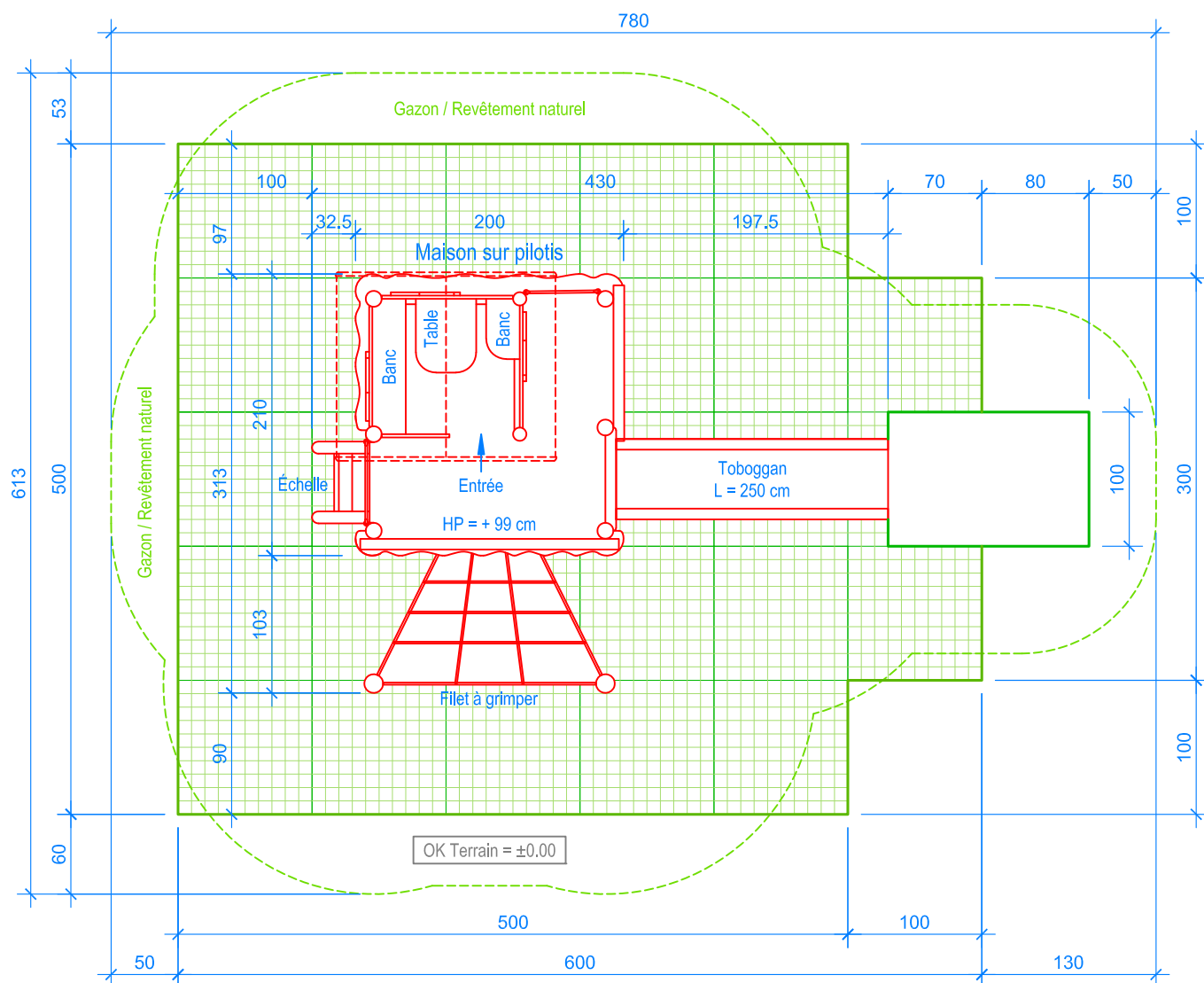
PLAN 1:50
