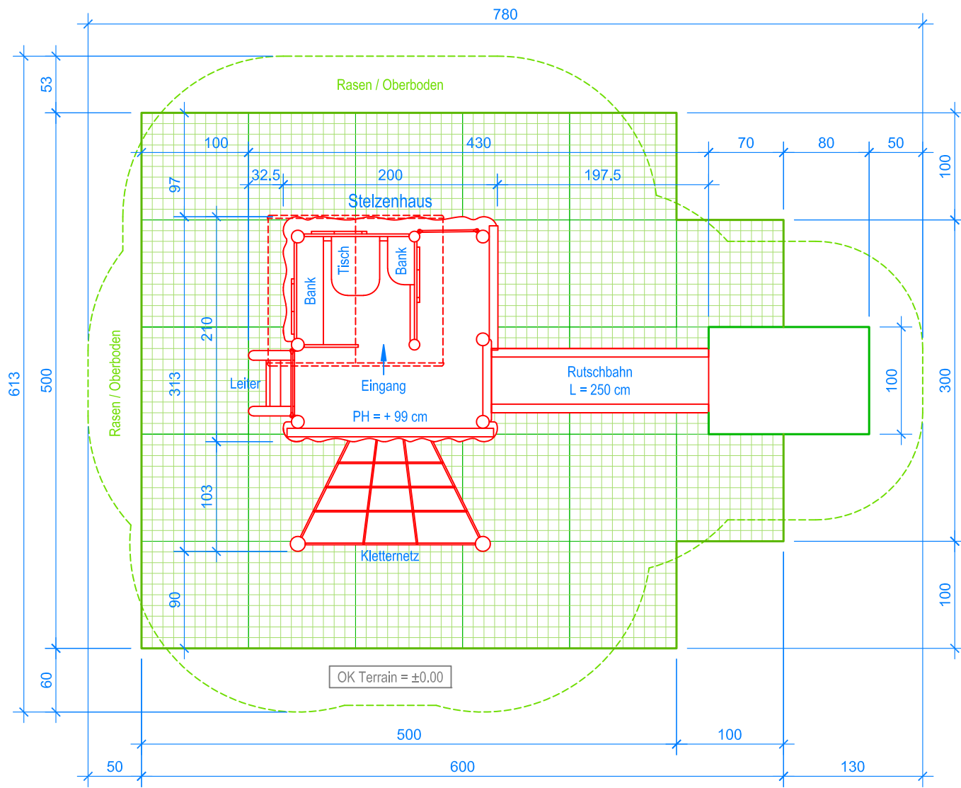
GRUNDRISS 1:50
