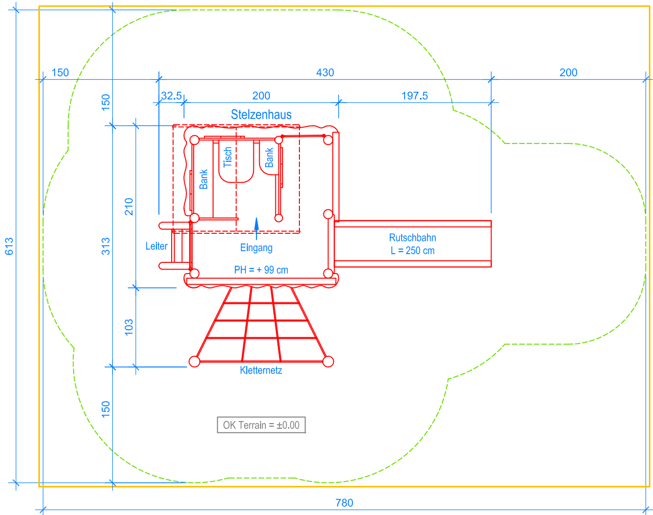
GRUNDRISS 1:50
