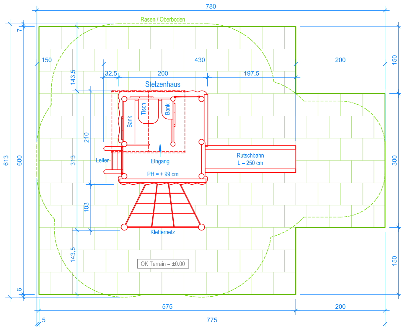
GRUNDRISS 1:50
