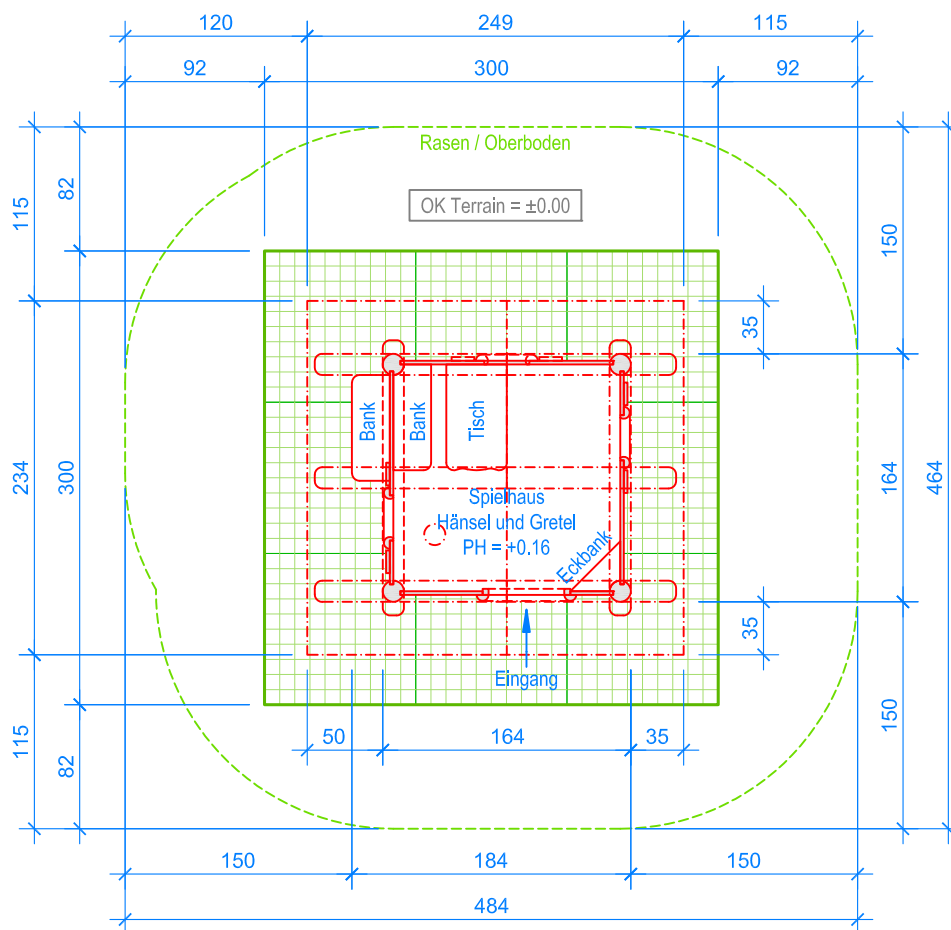
GRUNDRISS 1:50
