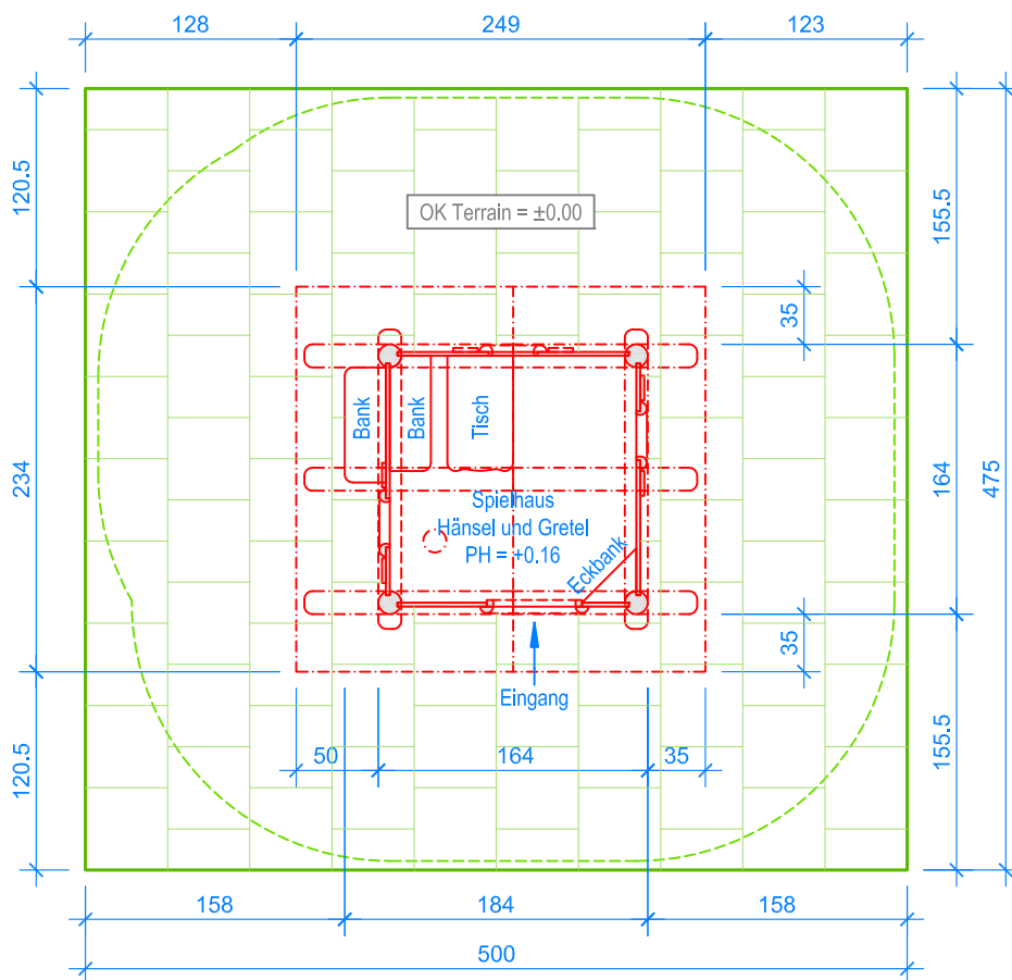
GRUNDRISS 1:50
