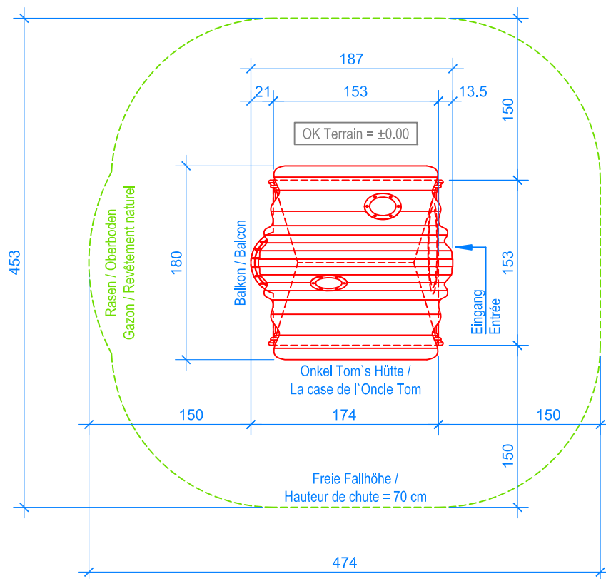
GRUNDRISS / PLAN 1:50
