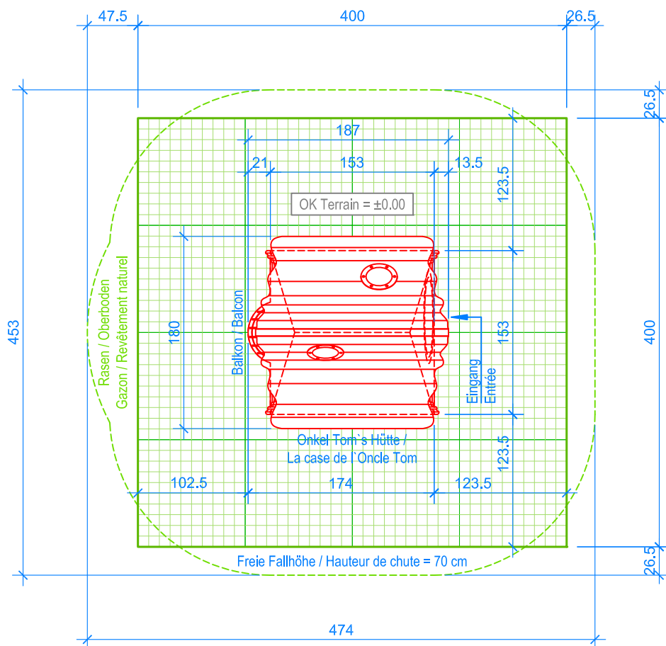
GRUNDRISS / PLAN 1:50
