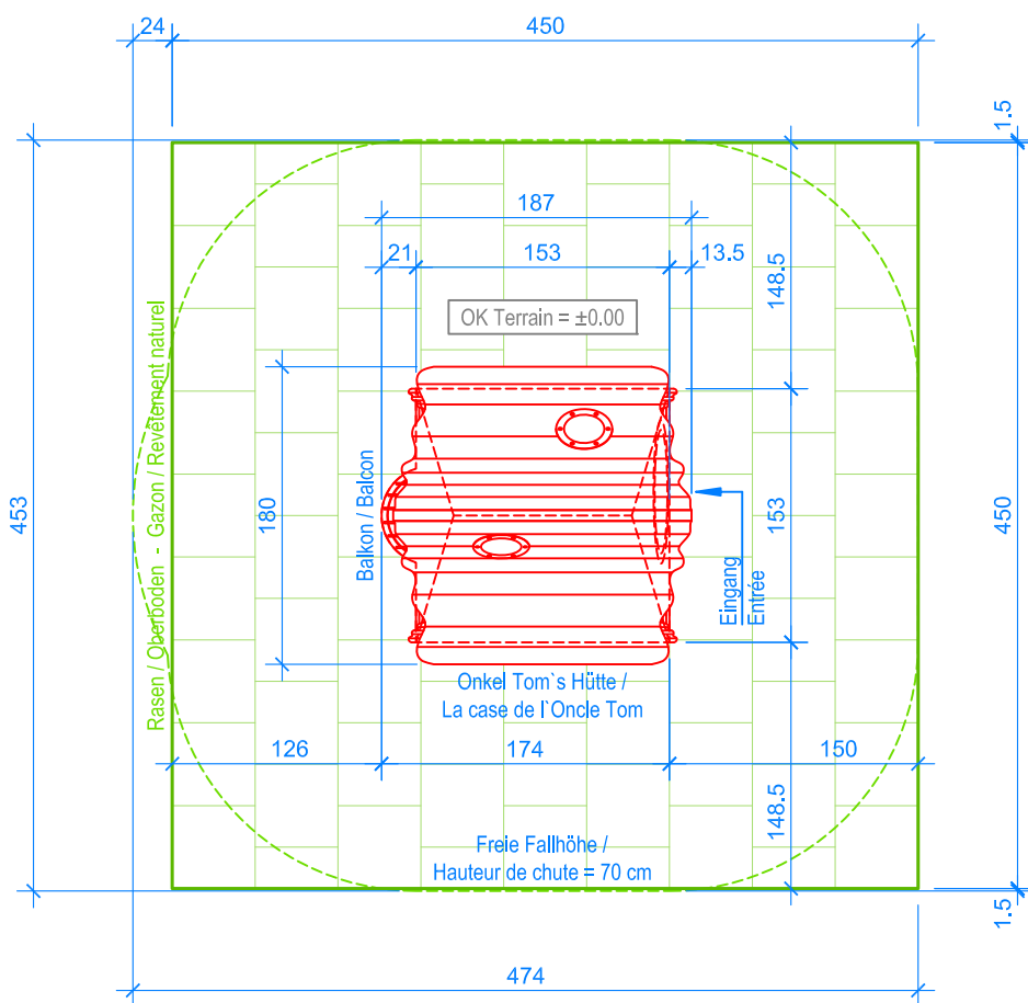
GRUNDRISS / PLAN 1:50
