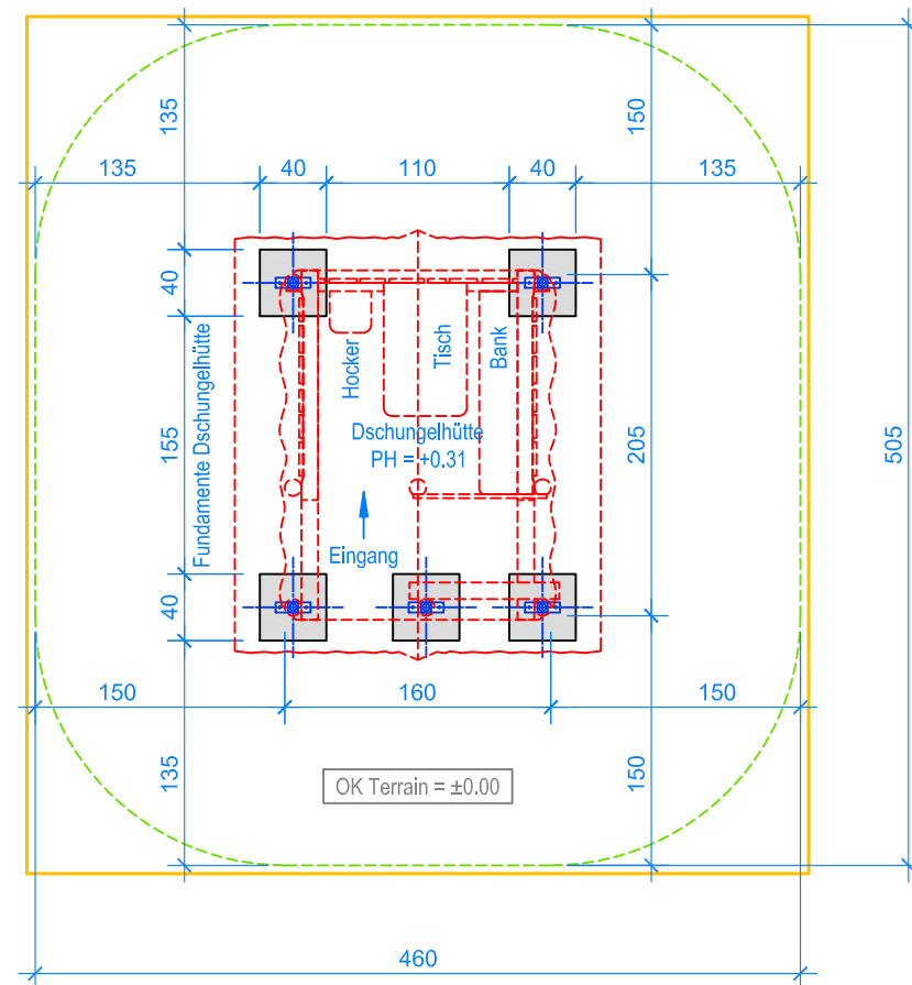
GRUNDRISS 1:50
