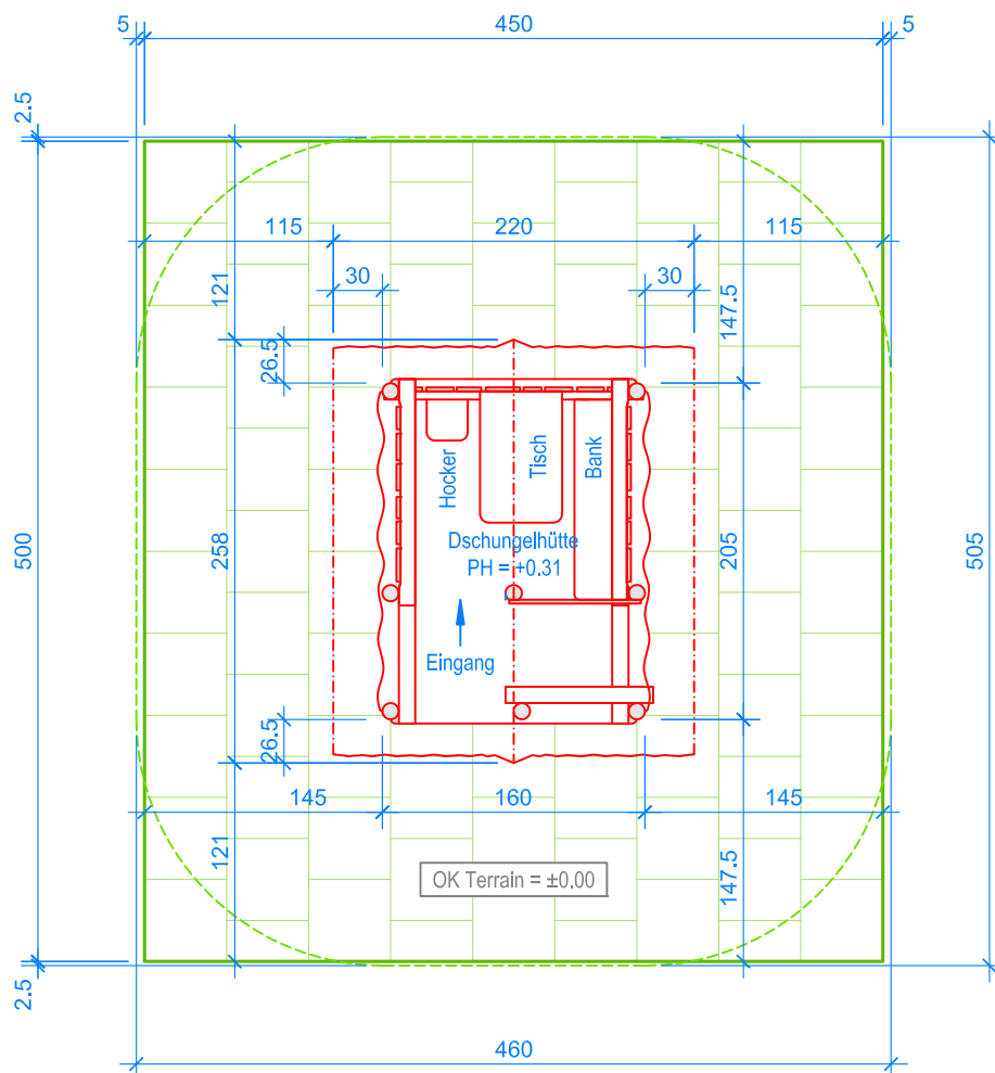
GRUNDRISS 1:50
