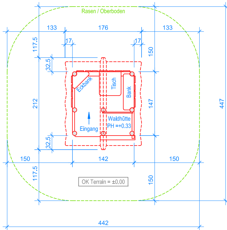
GRUNDRISS 1:50
