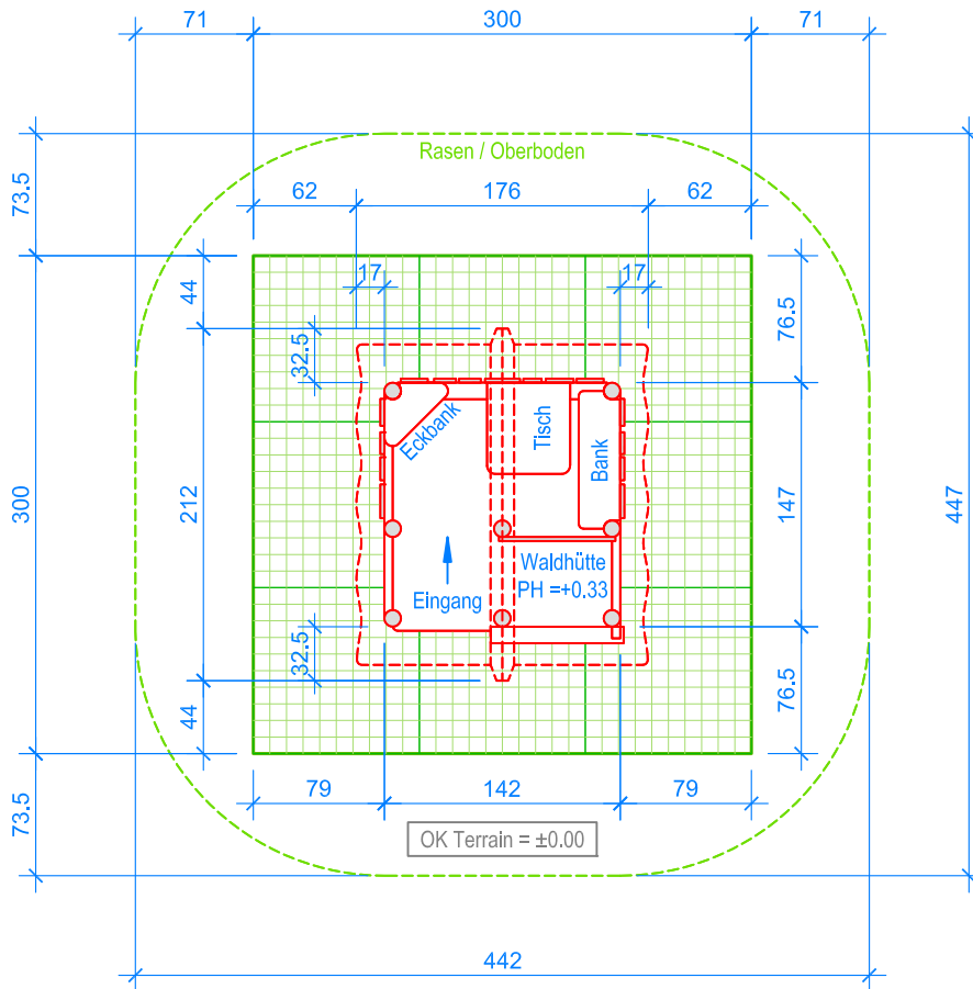
GRUNDRISS 1:50
