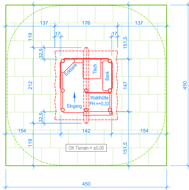
GRUNDRISS 1:50
