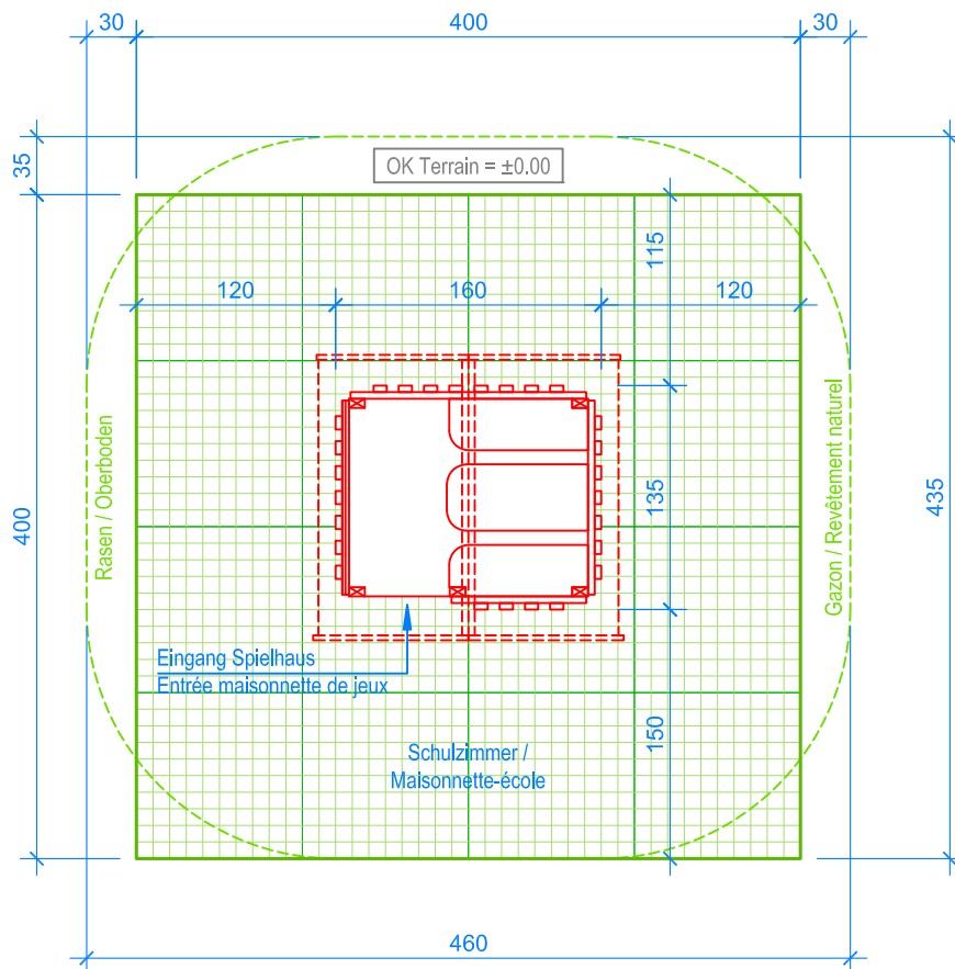
GRUNDRISS / PLAN 1:50
