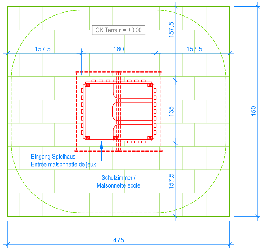
GRUNDRISS / PLAN 1:50
