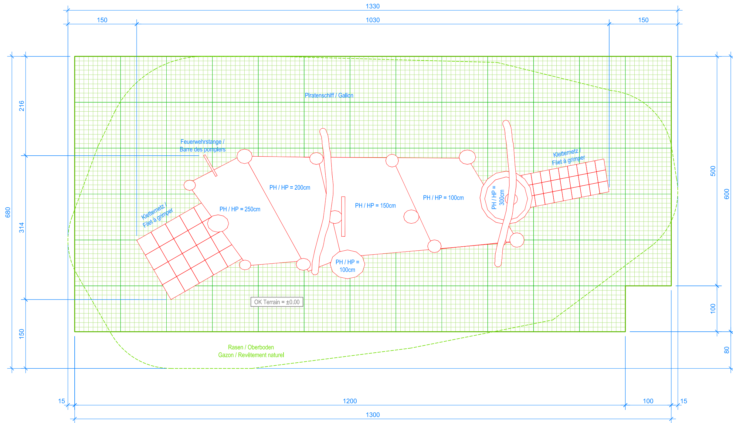
GRUNDRISS / PLAN 1:50
