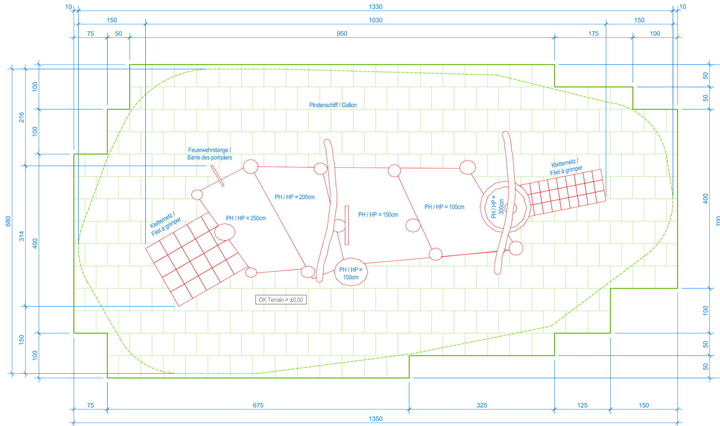
GRUNDRISS / PLAN 1:50
