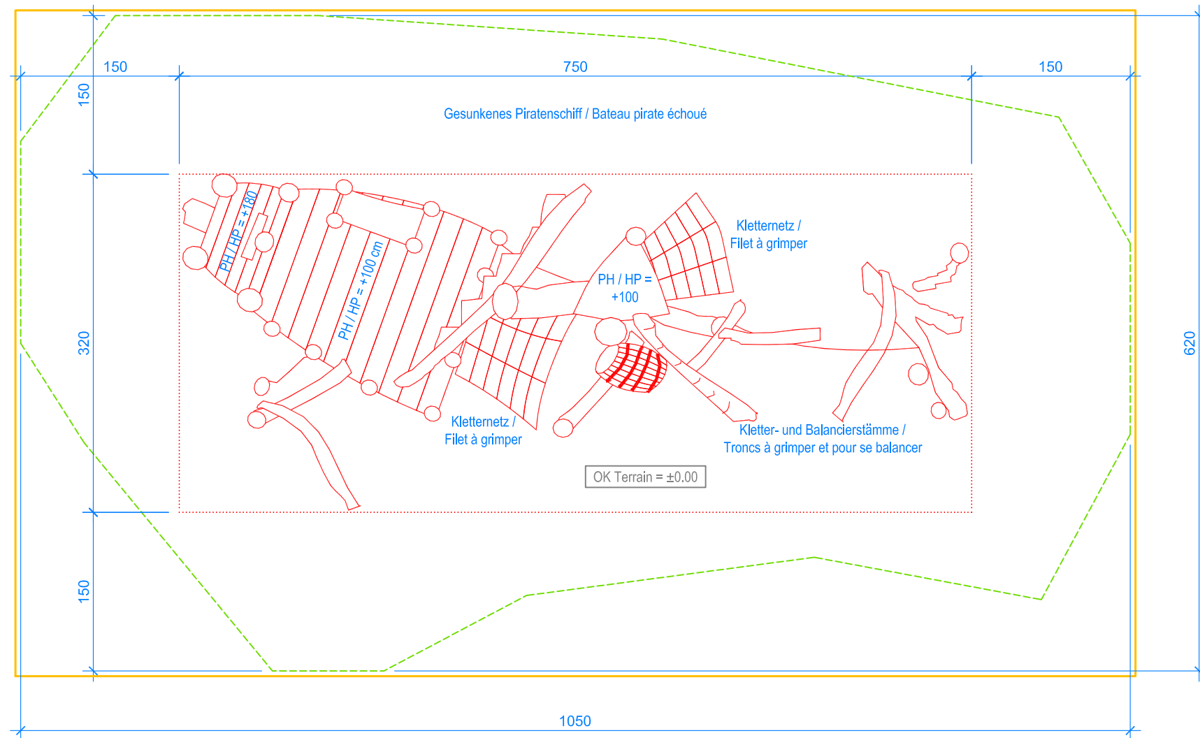
GRUNDRISS / PLAN 1:50
