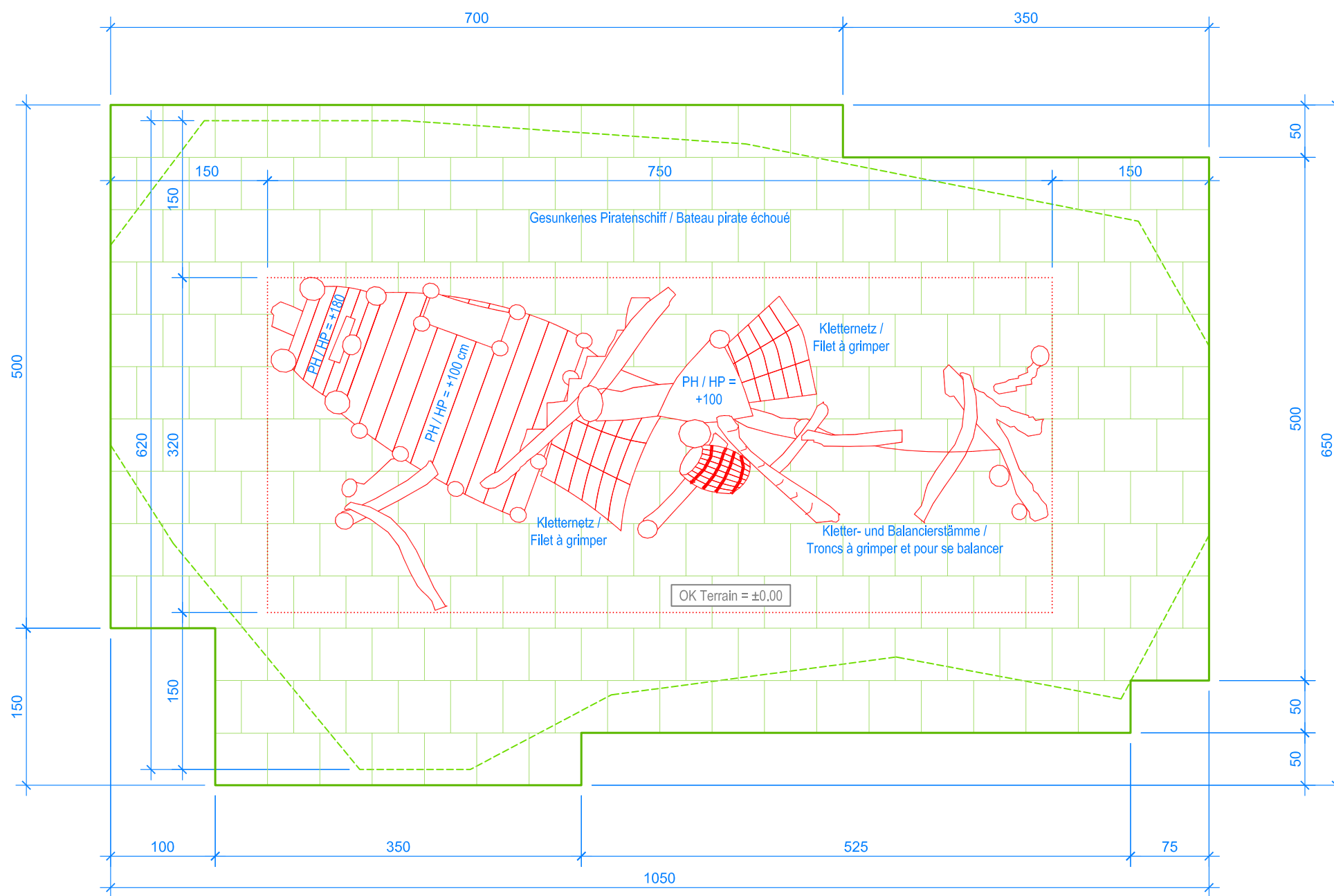
GRUNDRISS / PLAN 1:50
