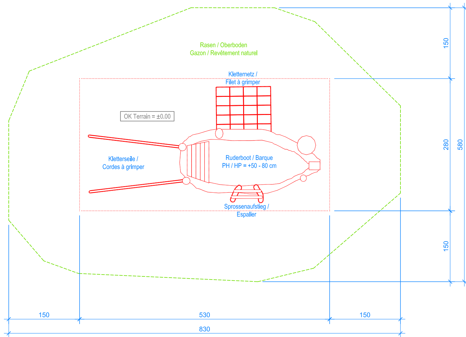
GRUNDRISS / PLAN 1:50
