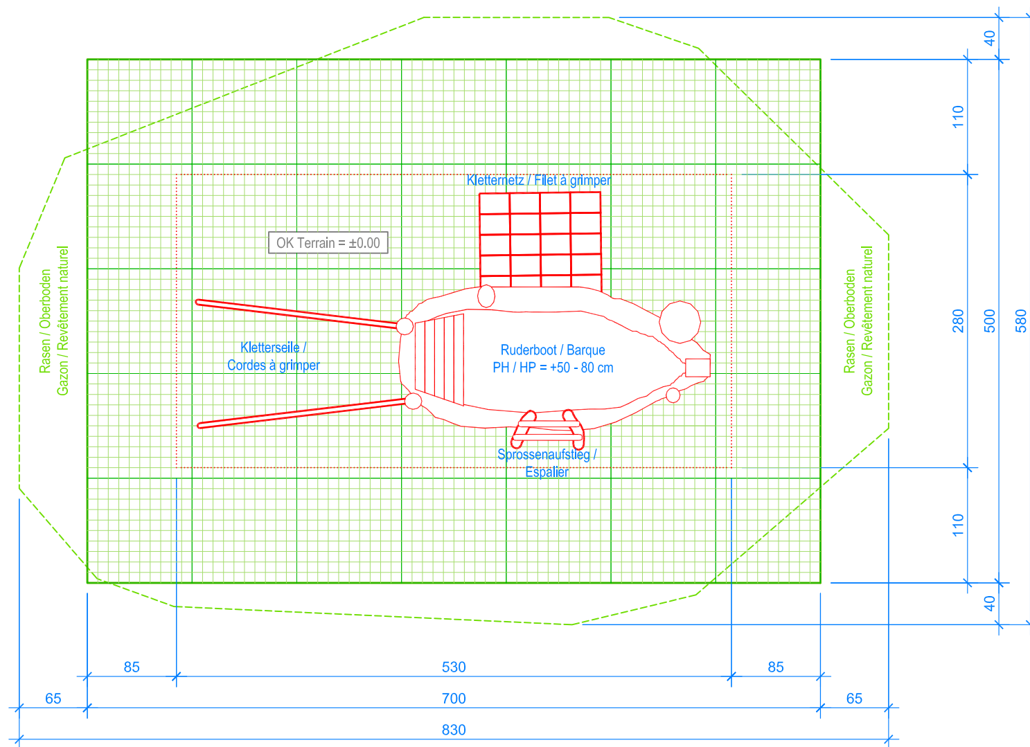
GRUNDRISS / PLAN 1:50
