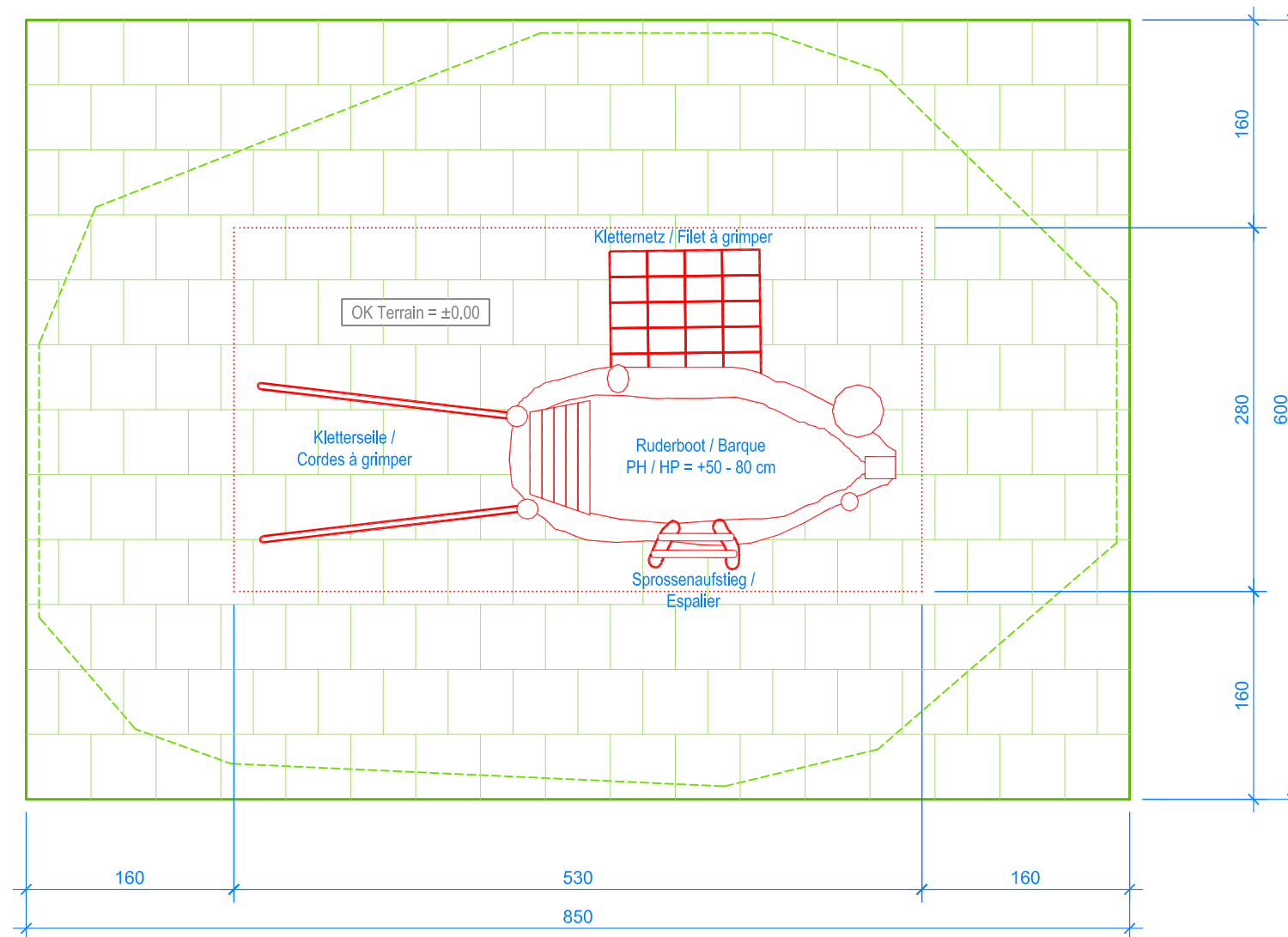
GRUNDRISS / PLAN 1:50
