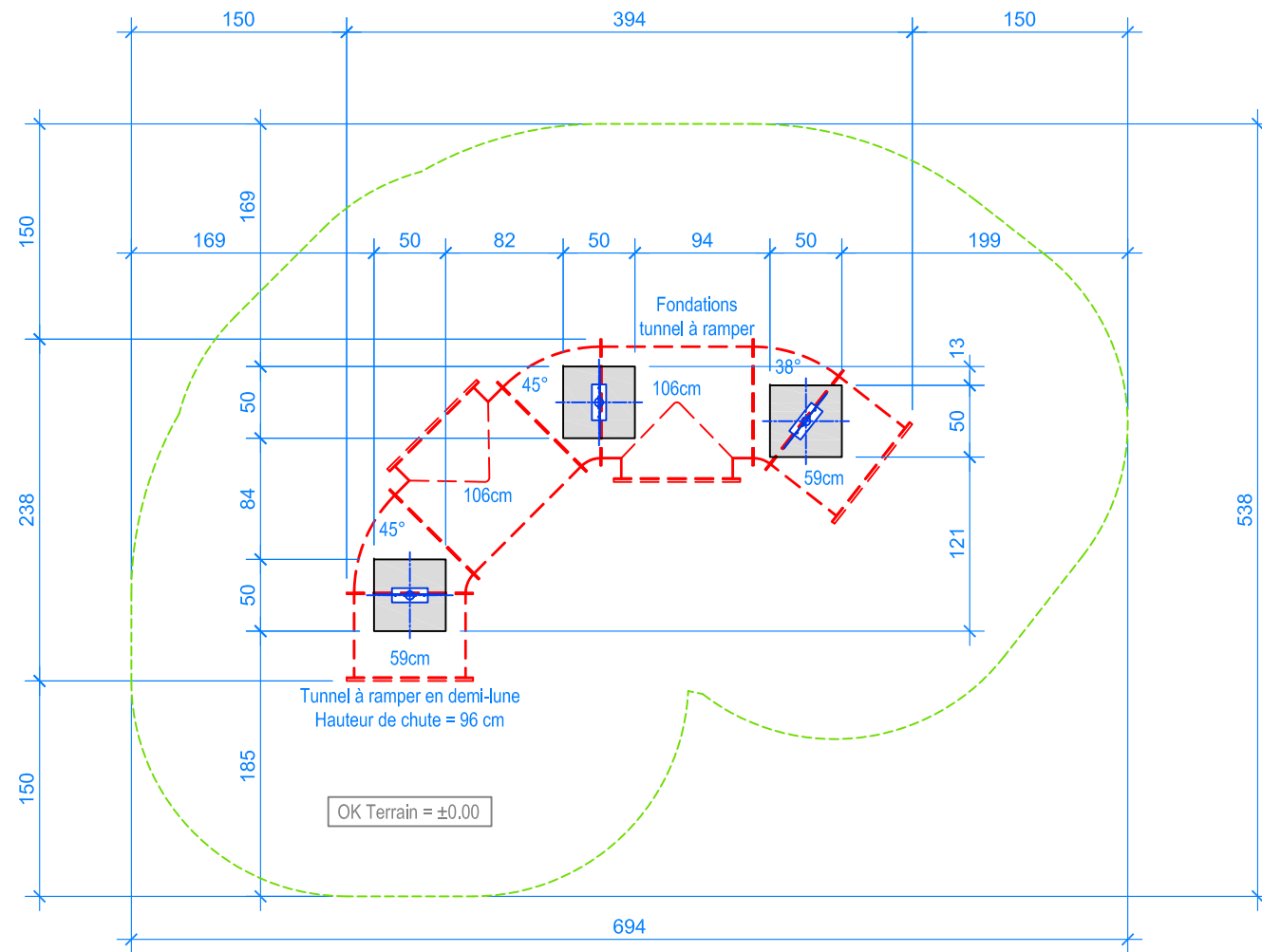
PLAN 1:50
