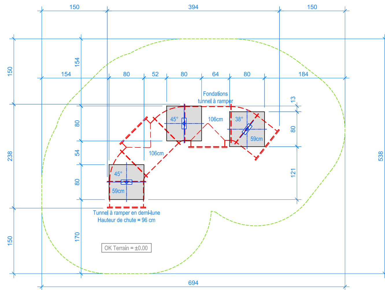
PLAN 1:50
