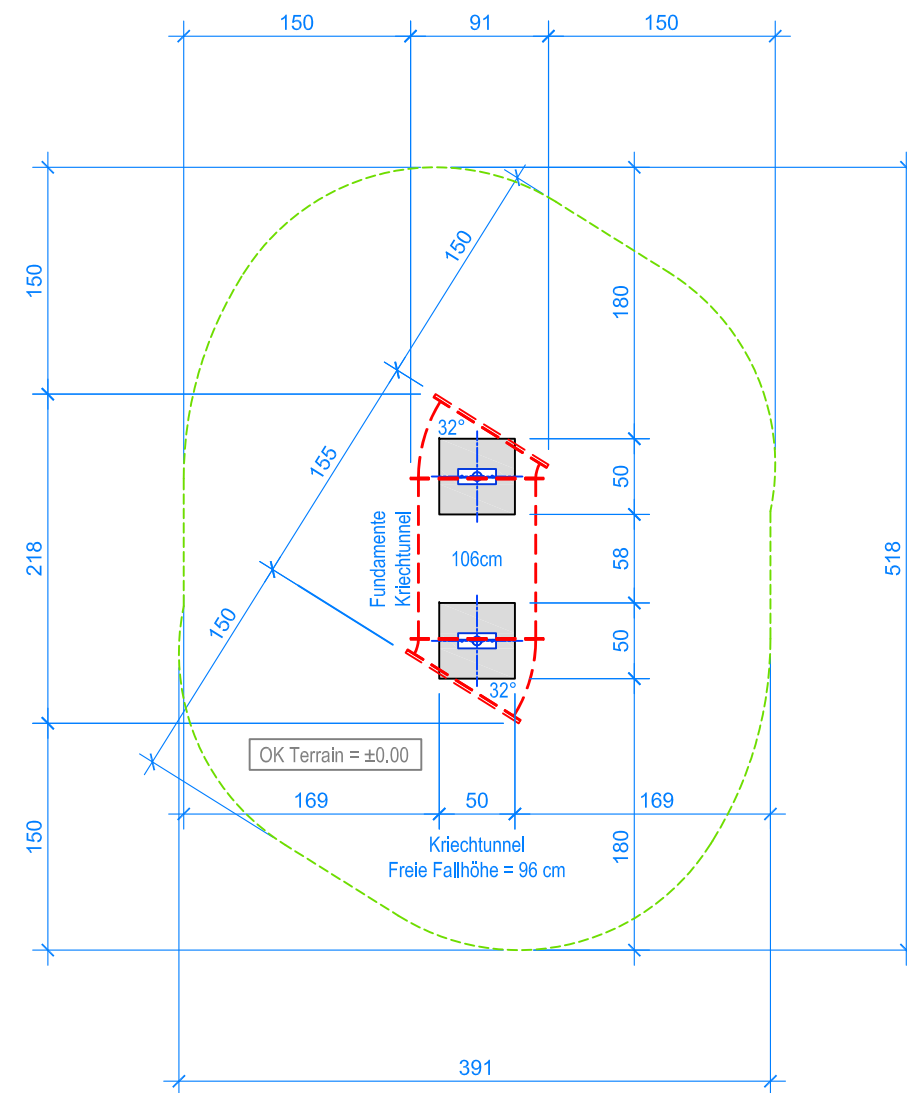
GRUNDRISS 1:50
