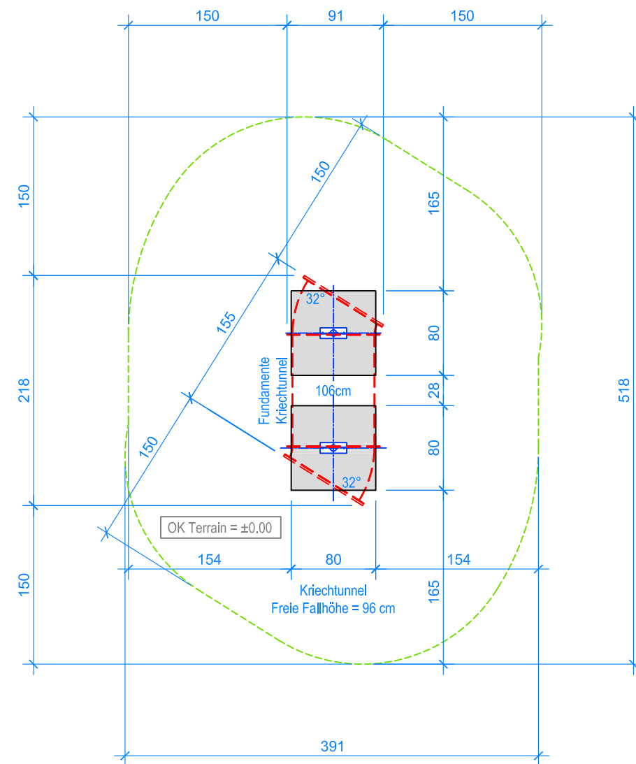
GRUNDRISS 1:50
