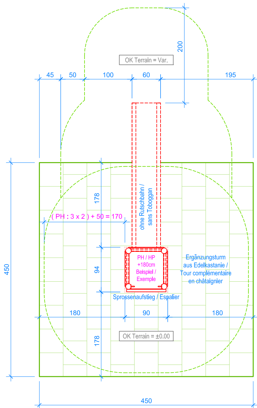
GRUNDRISS / PLAN 1:50
