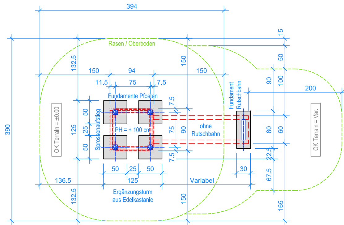
GRUNDRISS 1:50
