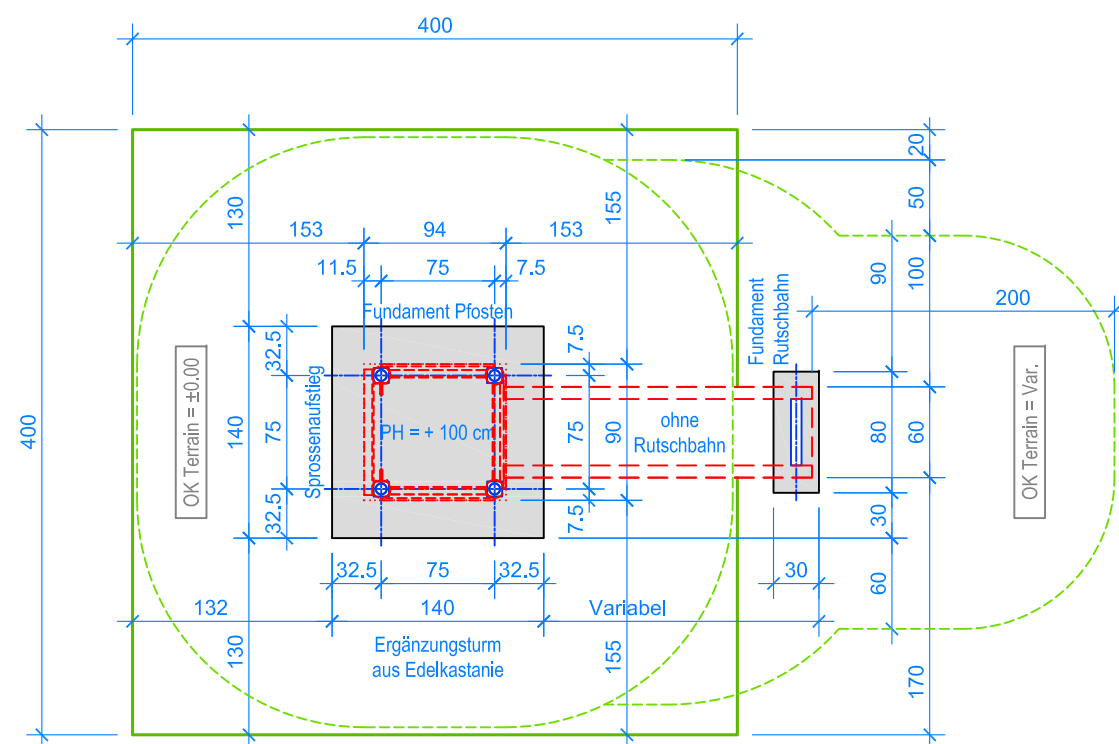
GRUNDRISS 1:50
