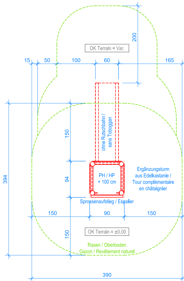
GRUNDRISS / PLAN 1:50
