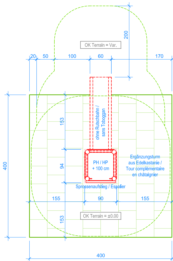
GRUNDRISS / PLAN 1:50
