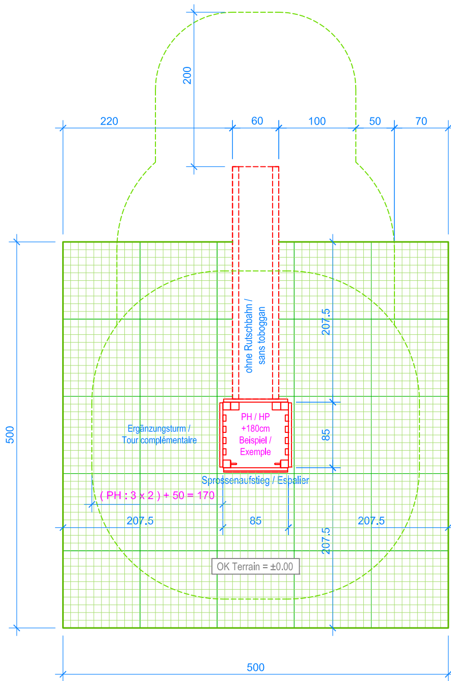
GRUNDRISS / PLAN 1:50
