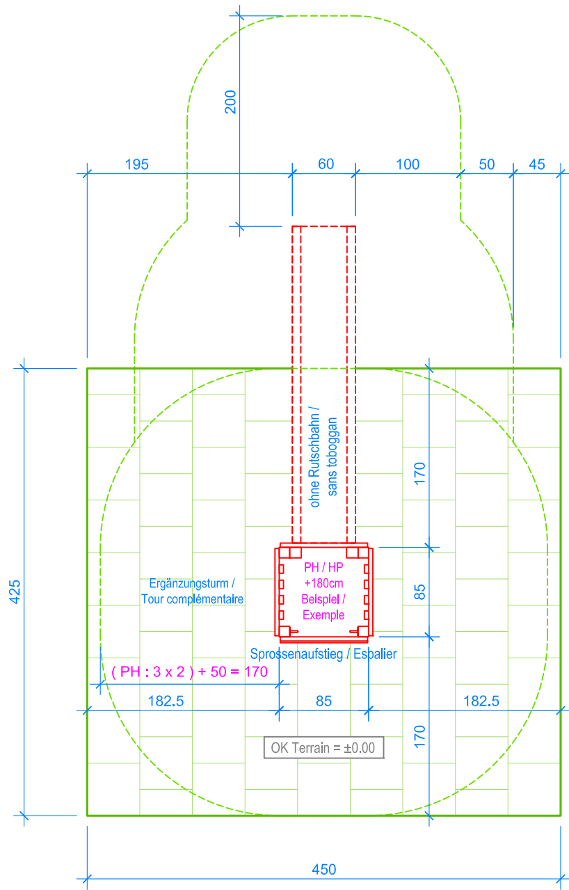
GRUNDRISS / PLAN 1:50
