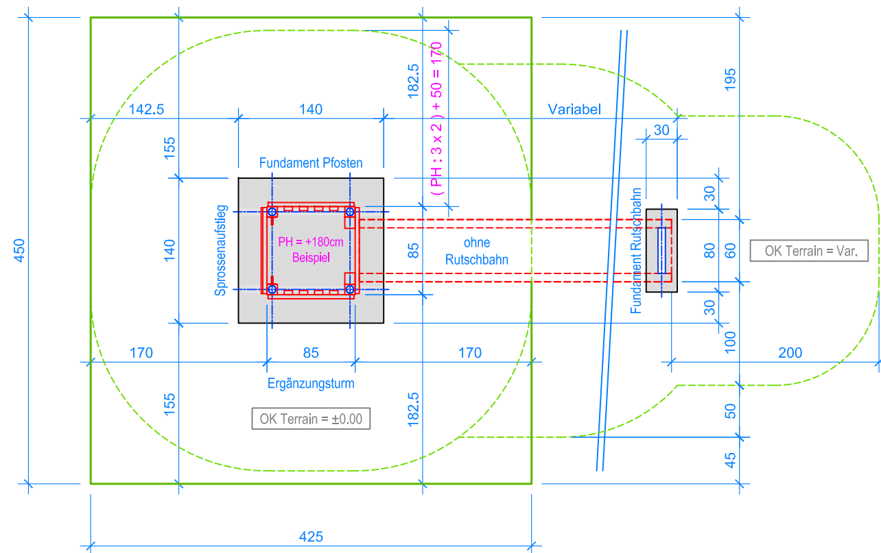
GRUNDRISS 1:50
