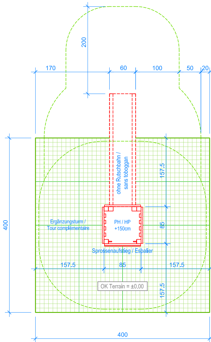
GRUNDRISS / PLAN 1:50
