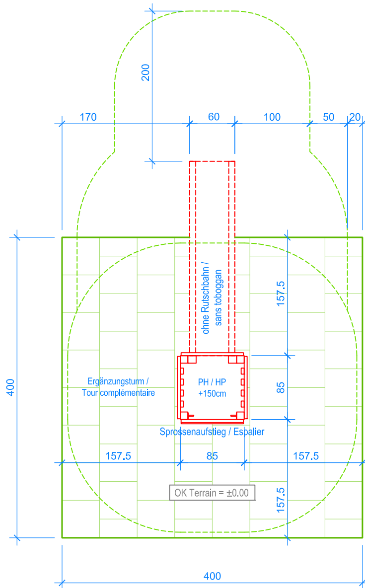
GRUNDRISS / PLAN 1:50
