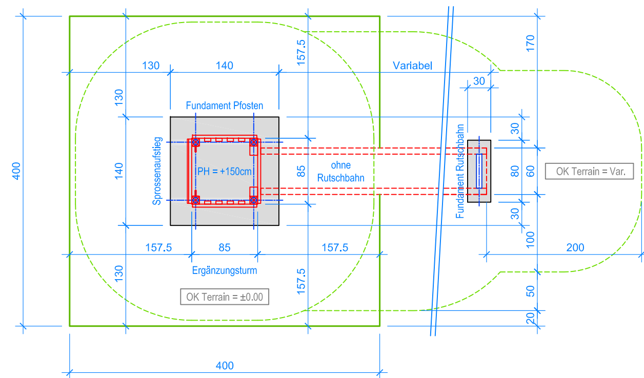
GRUNDRISS 1:50
