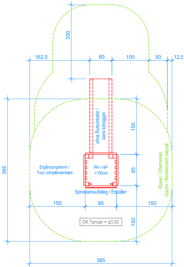
GRUNDRISS / PLAN 1:50
