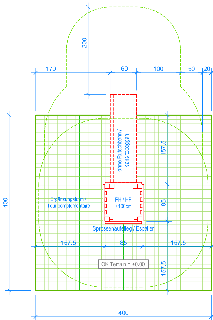
GRUNDRISS / PLAN 1:50
